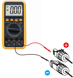
图5.15 万用表测量
